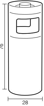
1615. NOX POSACENERE DA TERRA CON CESTINO GETTACARTE E VASCHETTA CON COPERCHIO AD ANELLO
