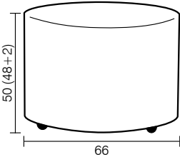
1686. NOX FLORA FIORIERA SU RUOTE PLANTER ON CASTORS Ø 52 x h 45 cm (43+2 cm) - 7,2 Kg dia. 20.5" x h 17.75" (17"+0.75") - 7,2 Kg sottovaso interno Ø 46,5 cm internal saucer dia. 18.25"
