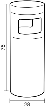
1613. NOX POSACENERE DA TERRA CON CESTINO GETTACARTE
